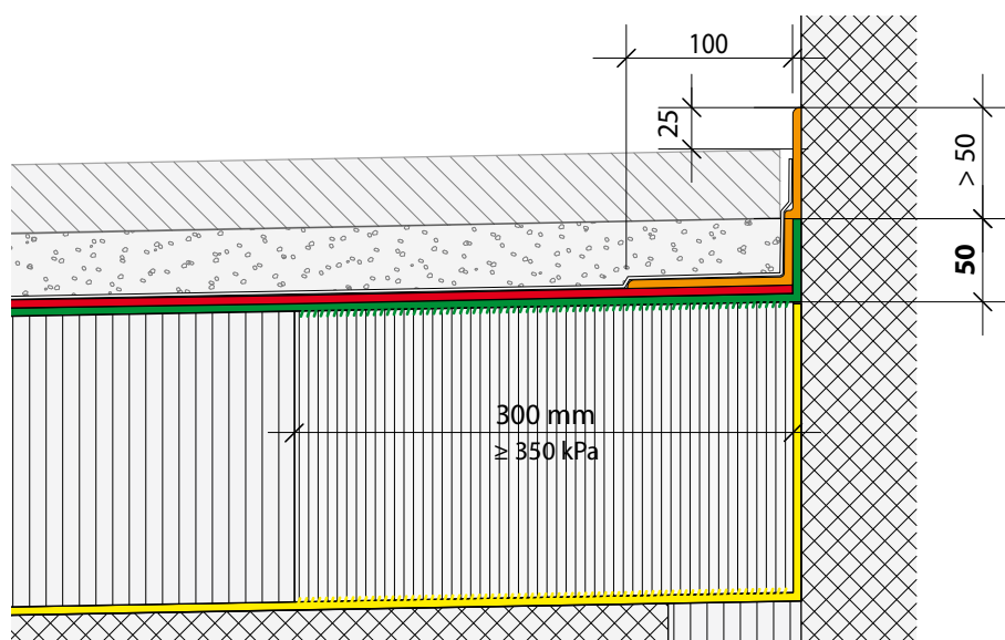
Fig. 1: Dans le cas de couches d'isolation thermique, il est nécessaire de fixer ou de coller une bande d'isolation sur le support d'au moins 300 mm de large et résistant à une pression d'au moins 350 kPa.
