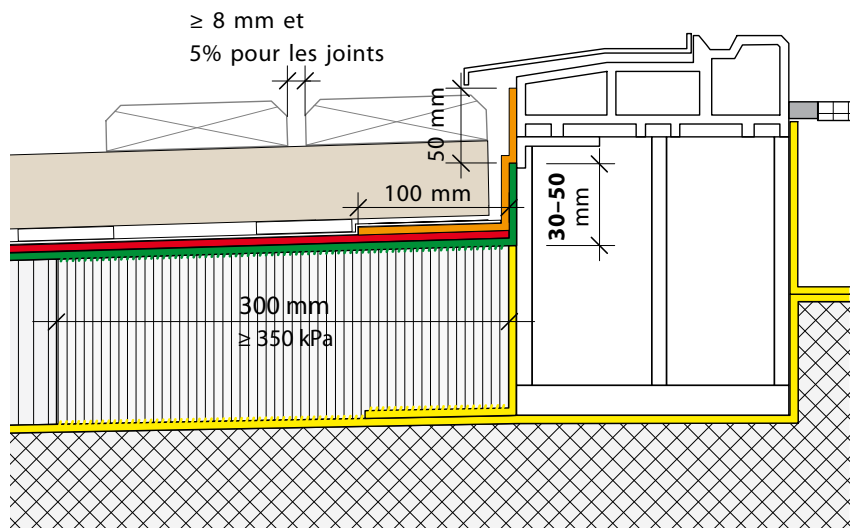
Fig. 4: Raccordement PL sur étanchement bitumineux à deux couches pour un raccords de seuil, hauteur du raccordement au-dessus de la couche d'usure inférieure à 60 mm. Réglementation d'exception de la norme SIA 271, observer le chiffre 5.2!
