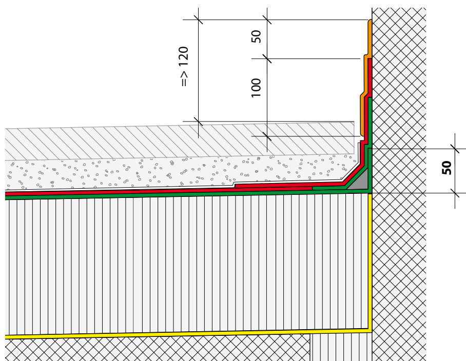
Fig. 2: Fermeture supérieure avec PL qui remplace la fermeture en tôle. Le relèvement bitumineux est réalisé de manière conventionnelle, avec coin et renfort d'angle.
