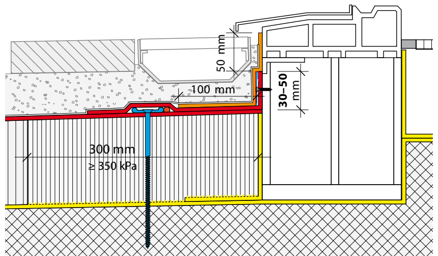
Fig. 5: Raccordement PL sur étanchement en lé synthétique pour un raccords de seuil, hauteur de raccordement au-dessus de la couche d'usure inférieure à 60 mm. Réglementation d'exception de la norme SIA 271, observer le chiffre 5.2!
