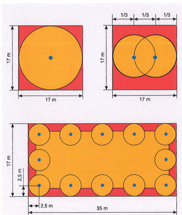
Fig. 22 à 24 Exemples de toits avec points d'ancrage individuels
