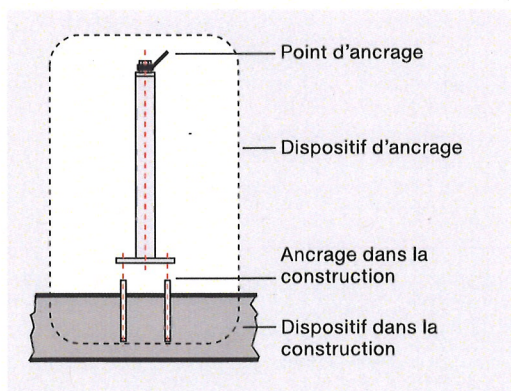
Fig. 7 Point d'ancrage individuel fixé dans la construction
